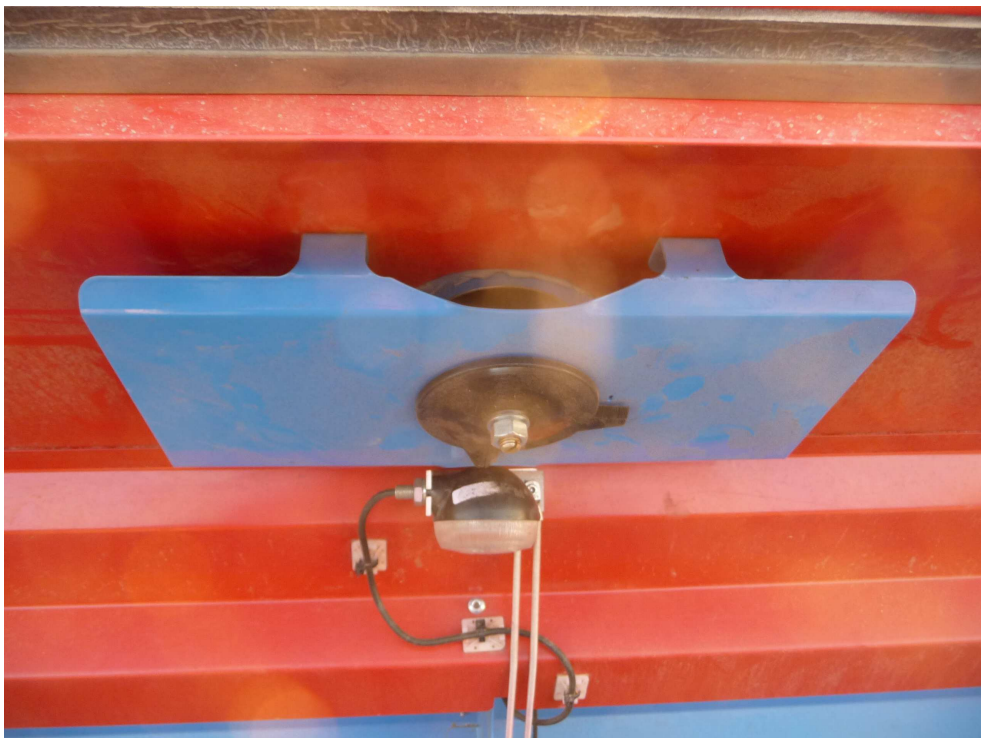
Zusatzrüstung pneumatisch Umladen - Rohrbogen mit Verteilblech im Sägerät, montiert im Sägeräte-Deckel
