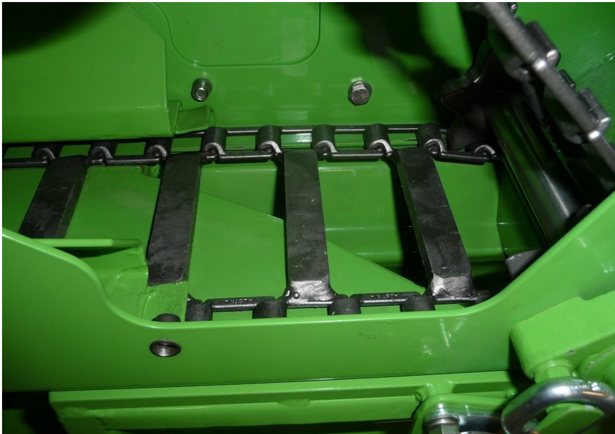
Aufbautank XEAT 2575 Inhalt 7500 Liter, Tankmaße innen 2,5 m Breite x 3,0 m Länge - mit 2 separat gesteuerten Kettendosierungen für Getreide oder Dünger → kontinuierliche Dosierung auch bei kleiner Ausbringmenge
